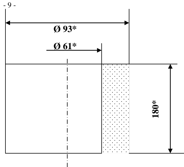
Рисунок 4 - Теплоизоляционная вставка
