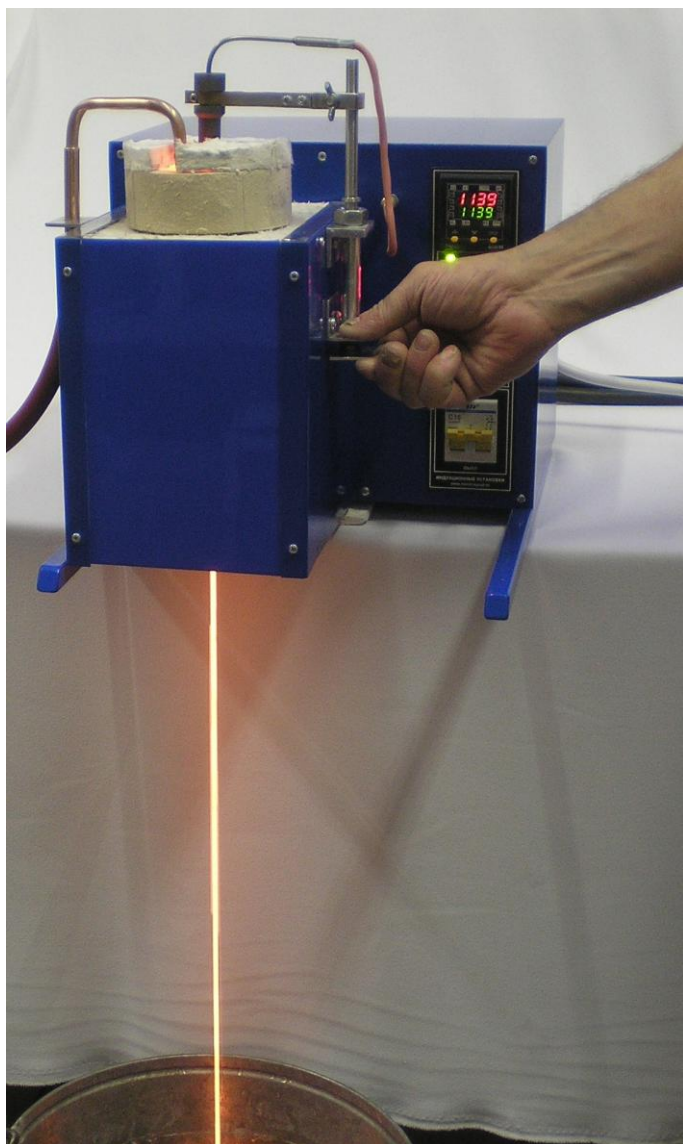
Рисунок 3 - донный розлив металла
